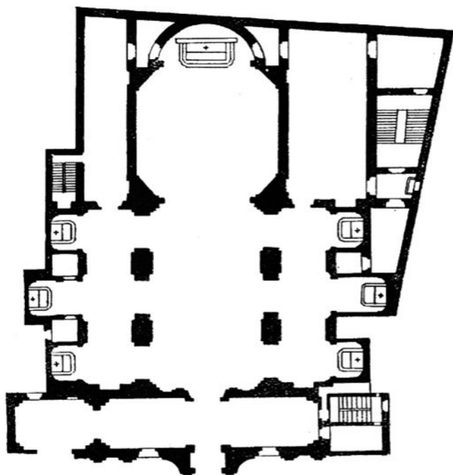
IL·LUSTRACIÓ 2. Església de la Santíssima Trinitat (1739-1743), Casa de la Missió de Montecitorio, a Roma, publicada a M. BOSI, «Una chiesa scomparsa», a B. BRIZZI, Album di Roma , Roma, Editori Romani Associati, 1980, p. 148.
